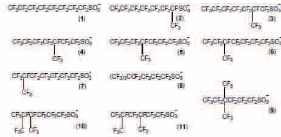
Figure 8 : Liste des 11 principaux isomères du PFOS (d'après Arsenault et al. (2008))
